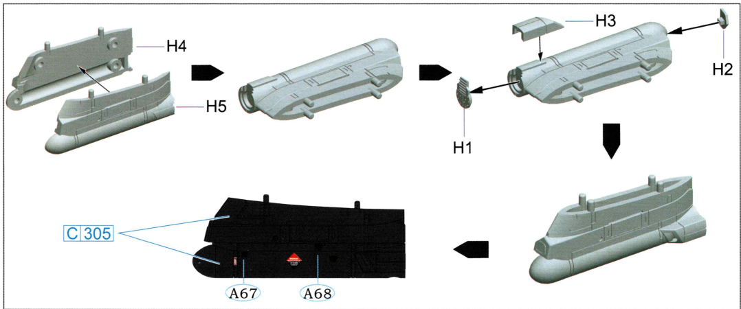
AN/AAQ-13低空导航吊舱 · AN/AAQ-13 Navigation Pod · AN/AAQ-13航法ポッド
