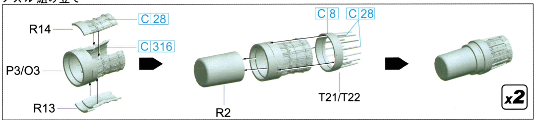
起飞降落状态組立 Gear Up Style Assemble 離陸状態組み立て
