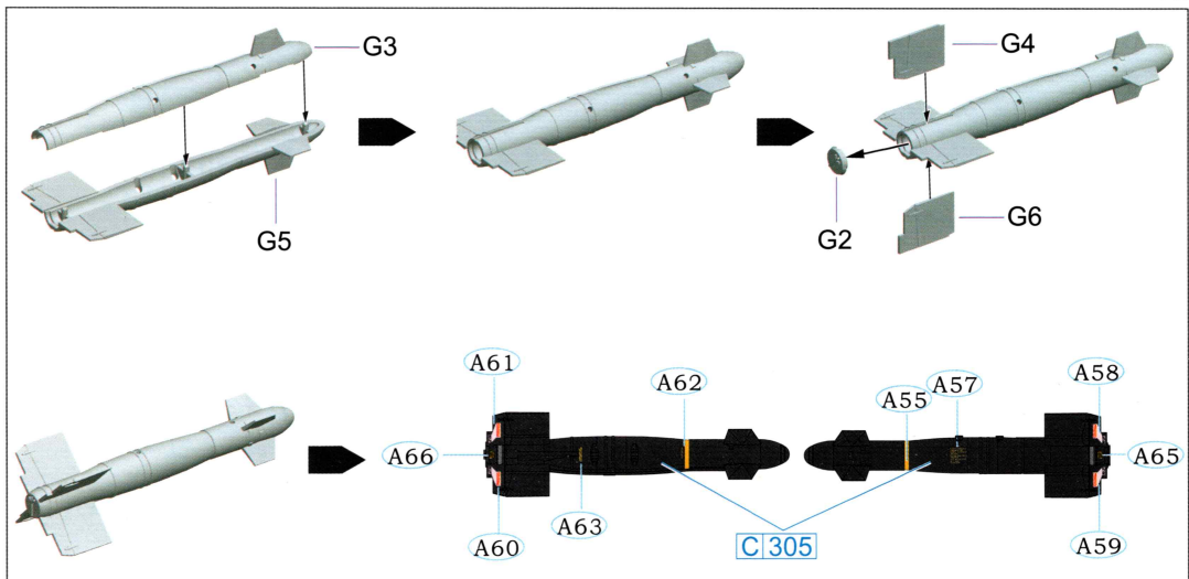
GBU-15电视制导炸弹 · GBU-15 TV-Guided Bomb · GBU-15誘導爆弾
