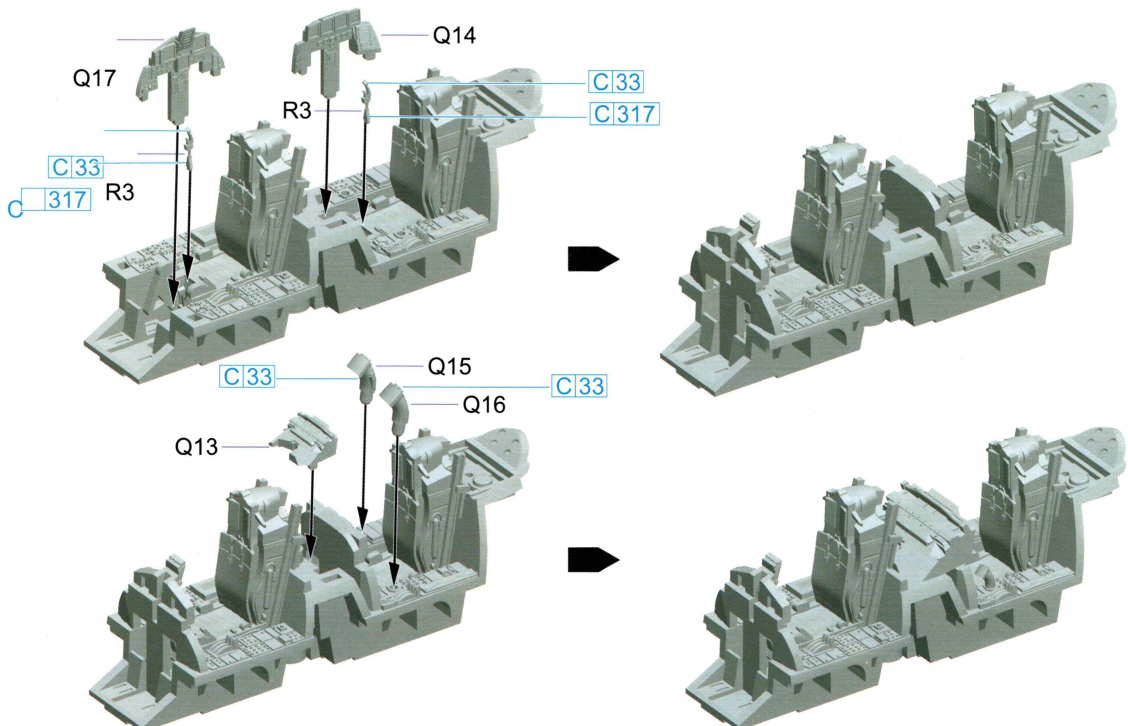
前仪表板 Front Instrument Panel 前にダッシュボード
