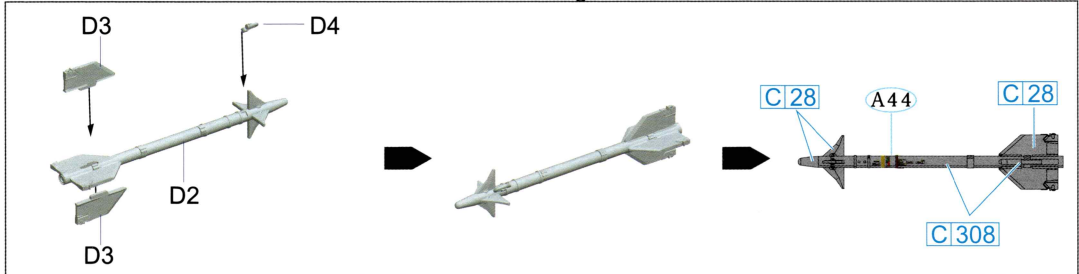
AIM-9L 响尾蛇格斗导弹 · AIM-9L "Sidewinder" Short Range Air-to-Air Missile · AIM-9L サイドワインダー X2
