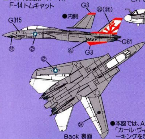
■F-14 TOMCAT VF-111 F-14 トムキャット
