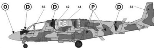
Расположение технических надписей для серийного вертолета Ka-50
