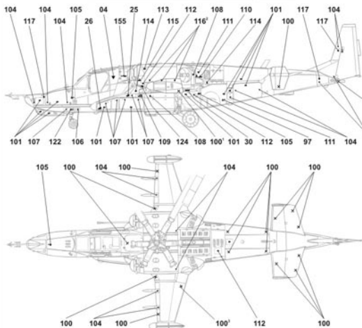
Расположение технических надписей для серийного вертолета Ka-50
