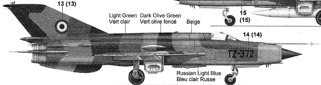
Mali Air Force MiG-21bis TZ-372, Bamako-Sénou AB 2008. MiG-21bis de la force aérienne du Mali, Sénou BA101. Roundels / Cocardes in six positions.
