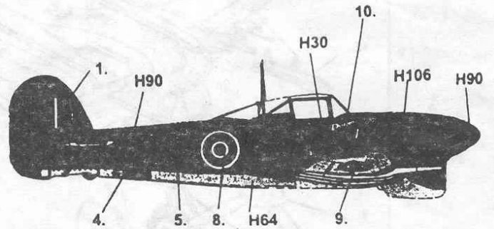
6) Тайфун Mk.Ib EL-C (DN421). 181 дивизион RAF.
