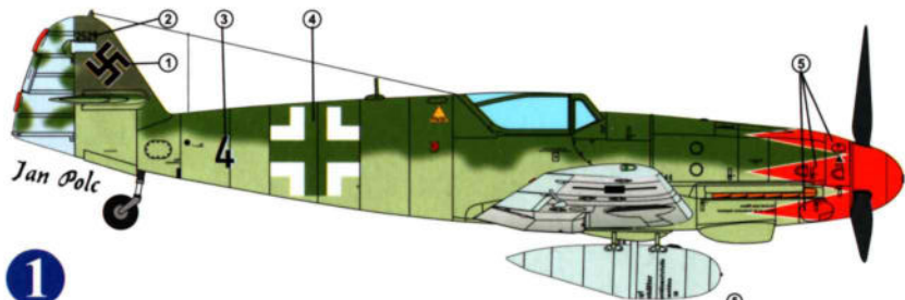
Bf 109K-4, W. Nr. 332529, „Black 4“, possibly of 1/JG 52, Deutsch Brod, Protektorat Böhmen und Mähren, April 1945.
