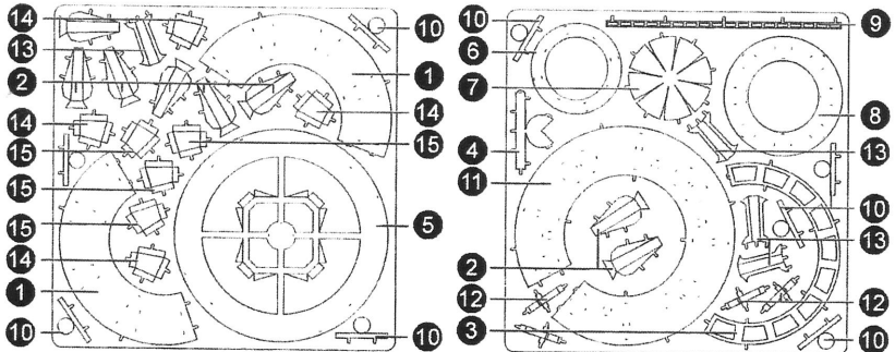
Schematic drawing of sheet metals (two pieces of sheet metal). 金屬片示意圖 (有2片金屬)
